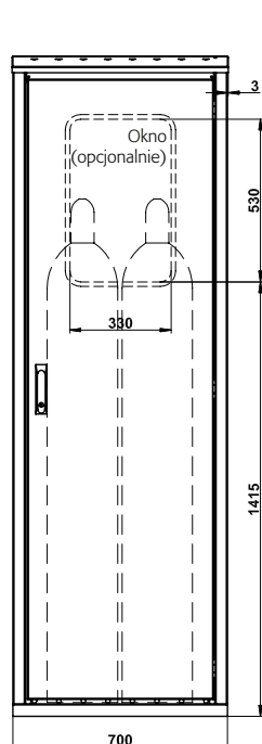
Model GOD.215.070.R - widok z przodu
