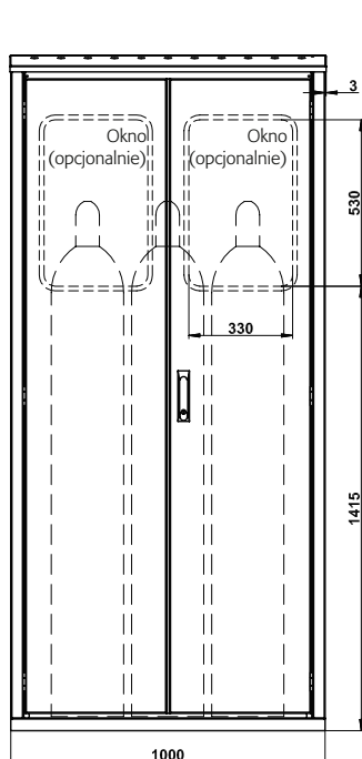
Model GOD.215.100 - widok z przodu
