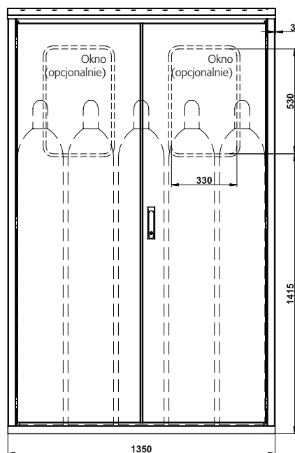
Model GOD.215.135 - widok z przodu
