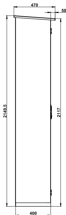
Model GOD.215.135 - widok z boku
